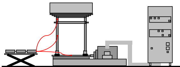
Gambar 6. Skema Rancangan Pengujian Model Struktur Rong-Rongan dengan Horizontal Slip Table
