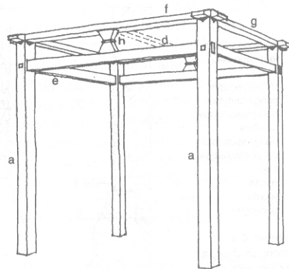
Gambar 4. Struktur Rong-Rongan dari dalam Rumah Joglo
