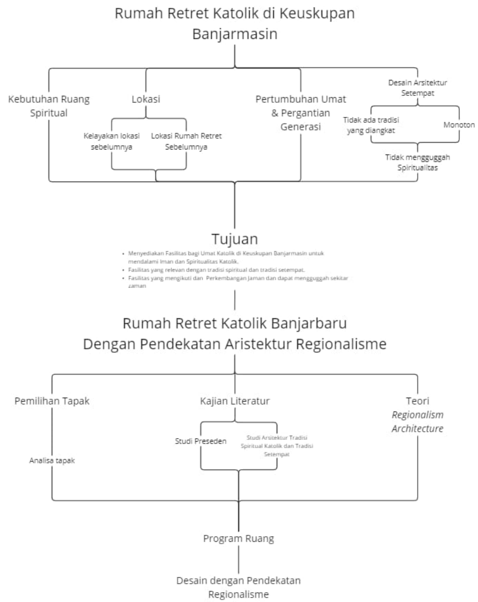
Gambar 1.3. Kerangka Berpikir
