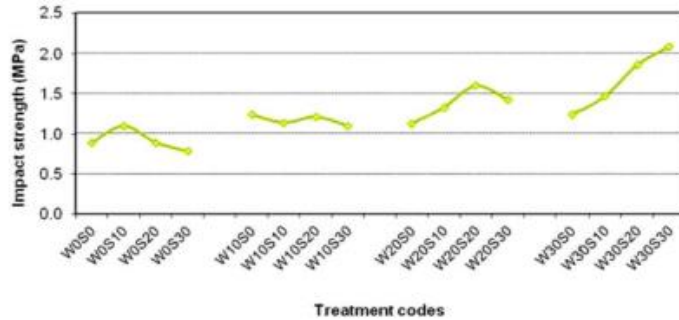
Gambar 2.6 Grafik perbandingan kekuatan impact pada komposit yang diisi PWF dan WSF
