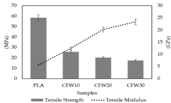
Gambar 2.5 Grafik uji tensile komposit PLA/CFW ( cotton fiber waste )
