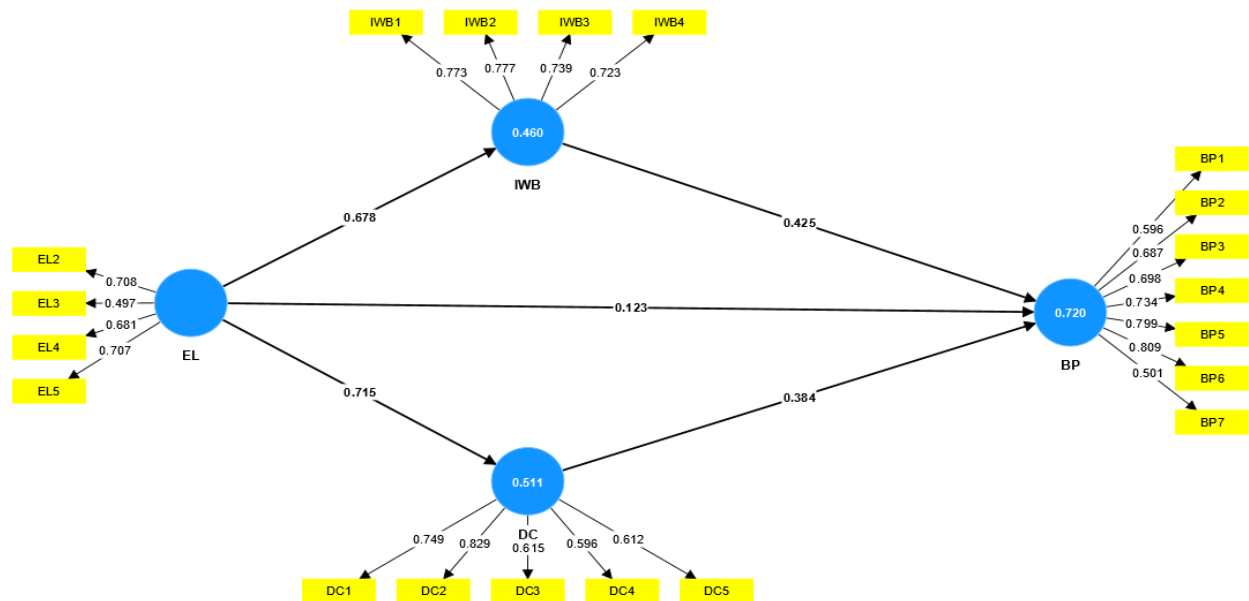
Lampiran 3J: Diagram Jalur PLS Algorithm Kedua
