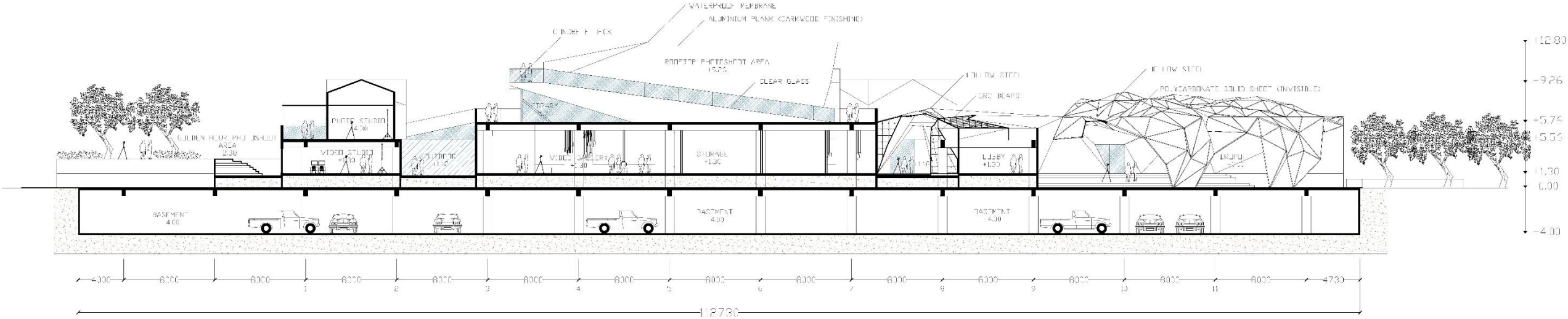
POTONGAN AA
