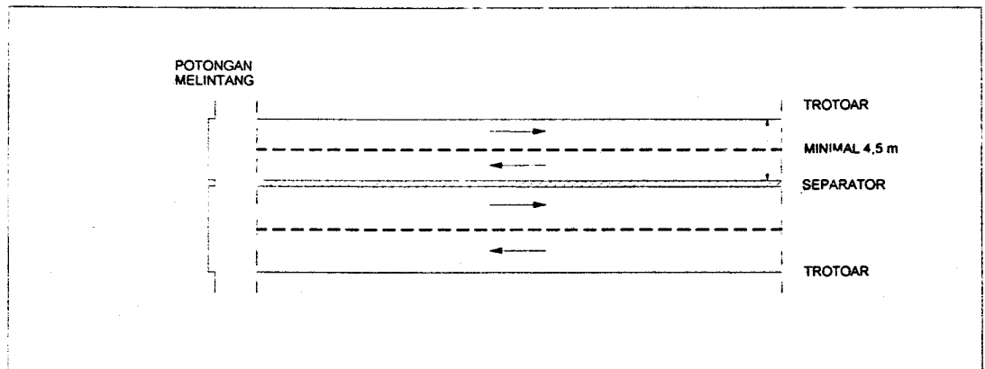
Gambar 5 Empat lajur dua jalur
