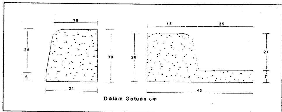
Gambar 7 Potongan melintang kereb
