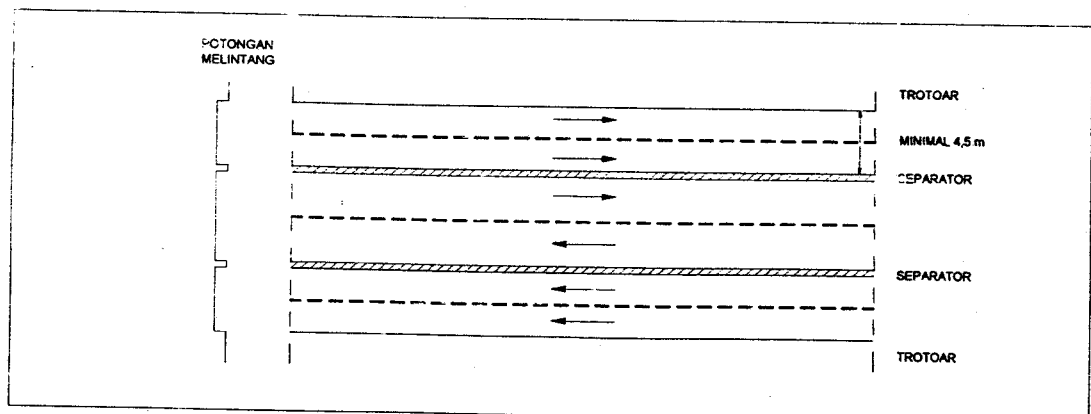
Gambar 3 Enam lajur dua arah tak terbagi
