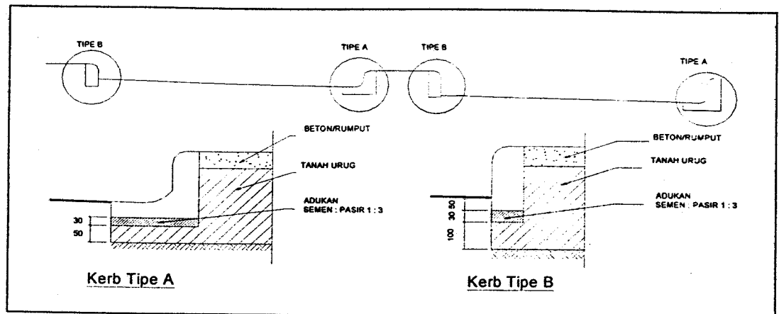
Gambar 6 Sisi luar separator yang dilengkapi kereb
