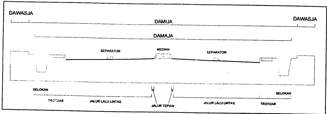
Gambar 1 Potongan melintang jalan dengan median
