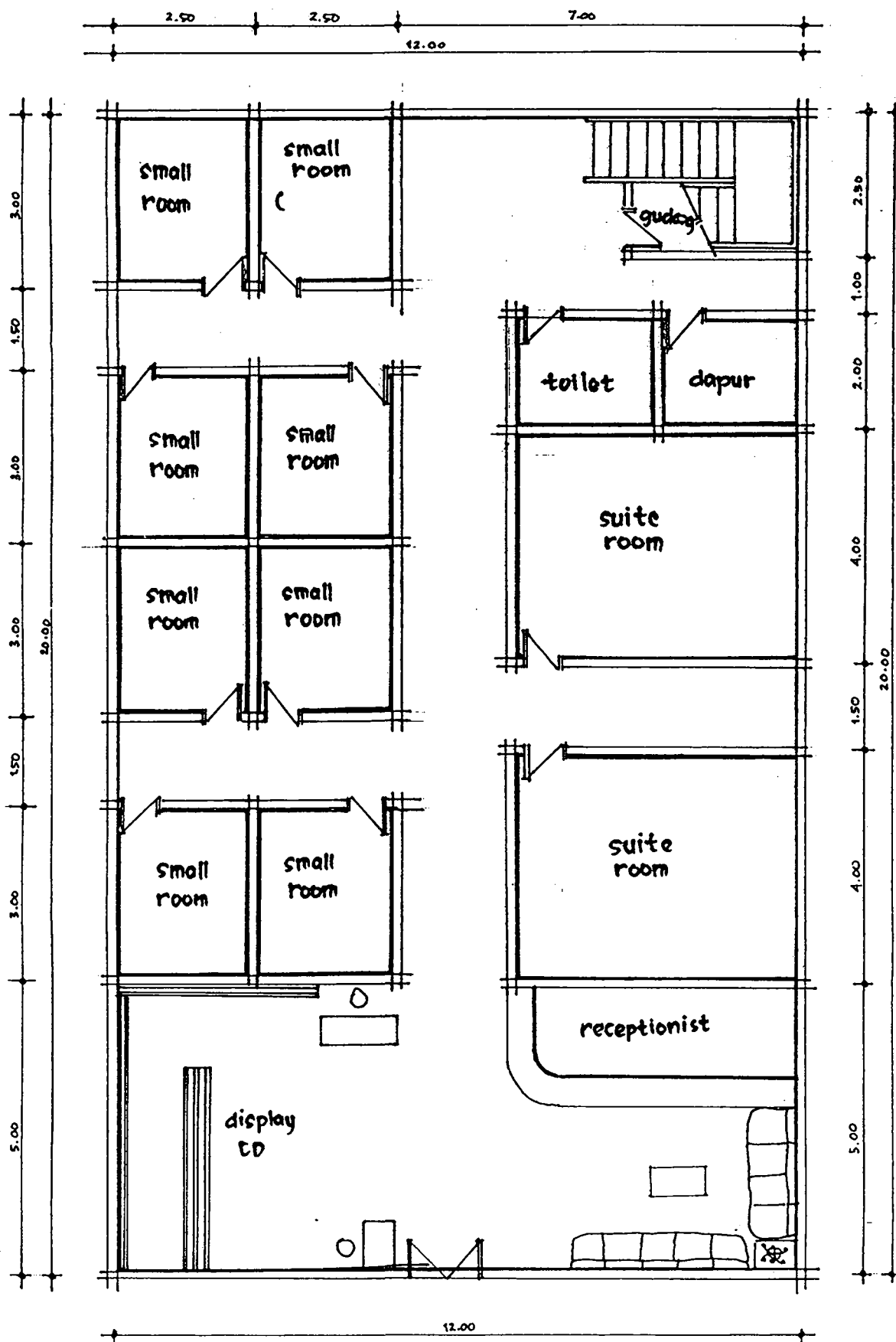
DENAH LT. 1 SKALA 1 : 100
