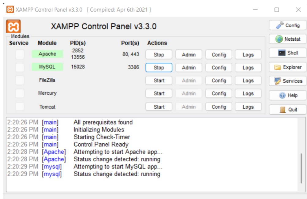
Gambar 4.1 Instalasi XAMPP
