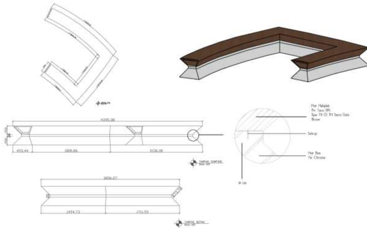
Gambar 7.13. Detail tempat duduk
