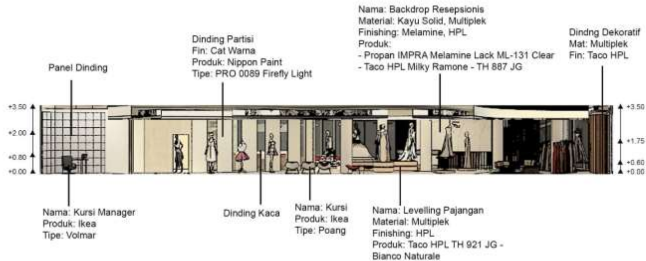
Gambar 7.20. Potongan C-C'
