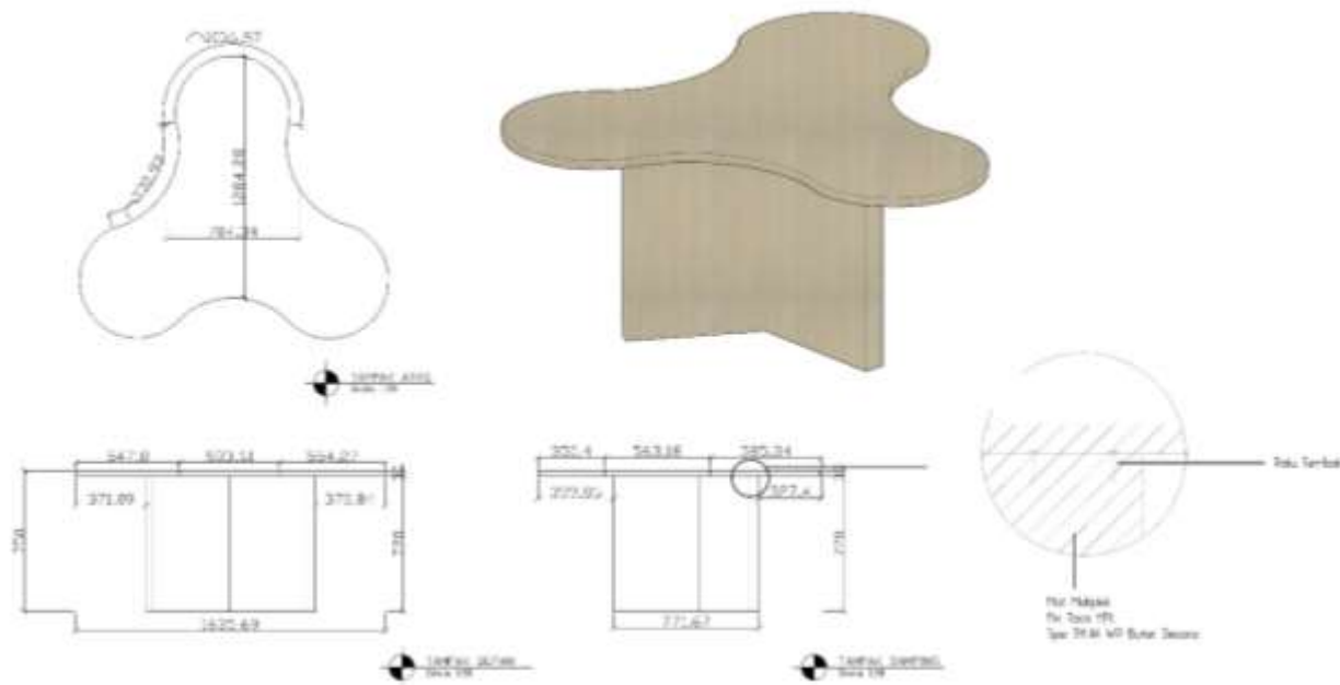
Gambar 7.14. Detail meja karyawan
