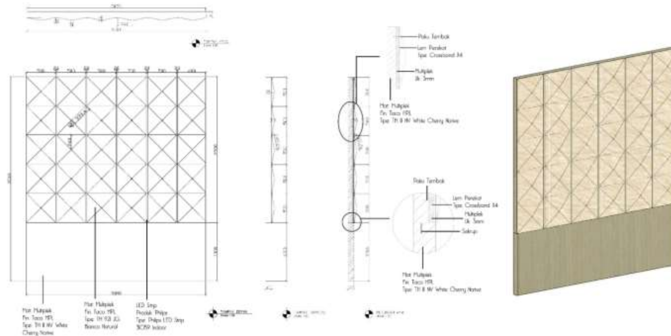
Gambar 7.7. Detail dinding dekoratif
