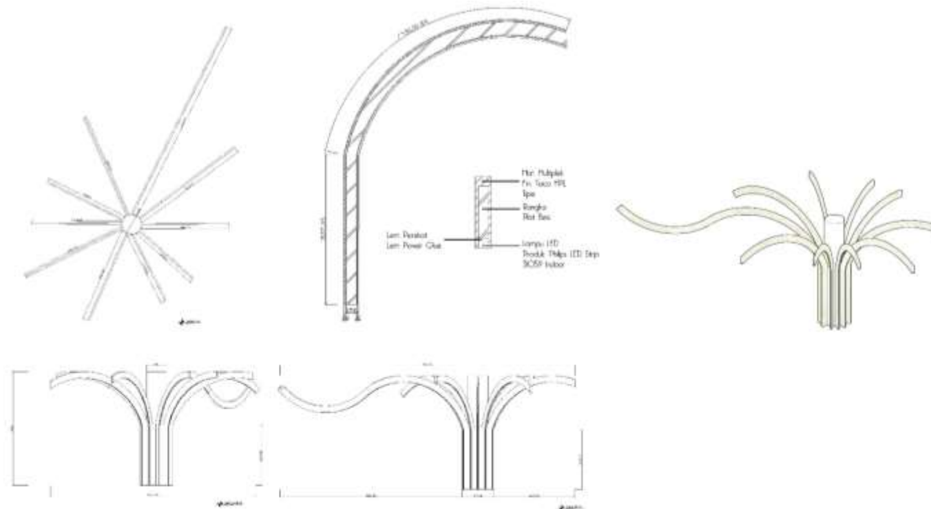
Gambar 7.9. Detail kolom dekoratif
