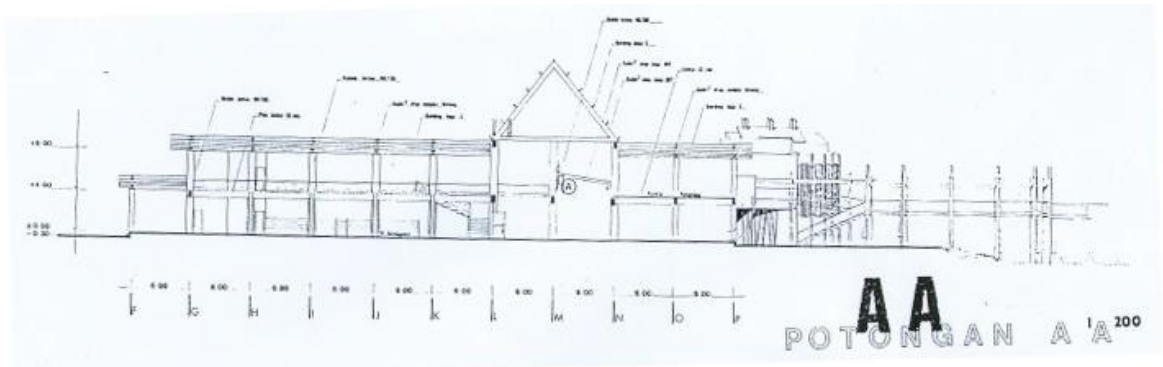
Gambar 3.4. Potongan A-A'
