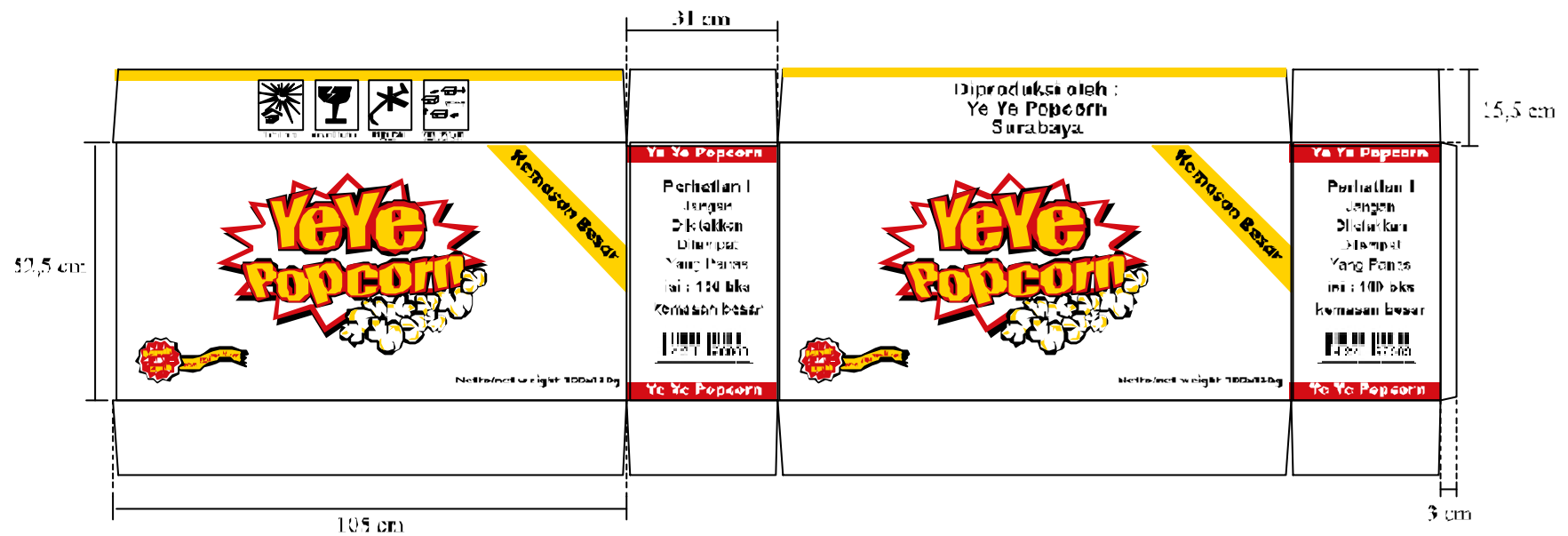
Gambar 6.3. Pattern Kemasan Sekunder Besar
