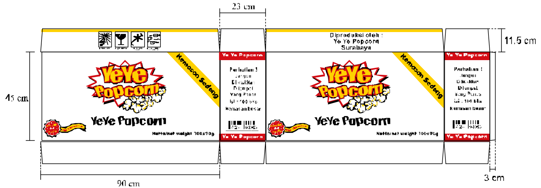
Gambar 6.9. Pattern Kemasan Sekunder Sedang
