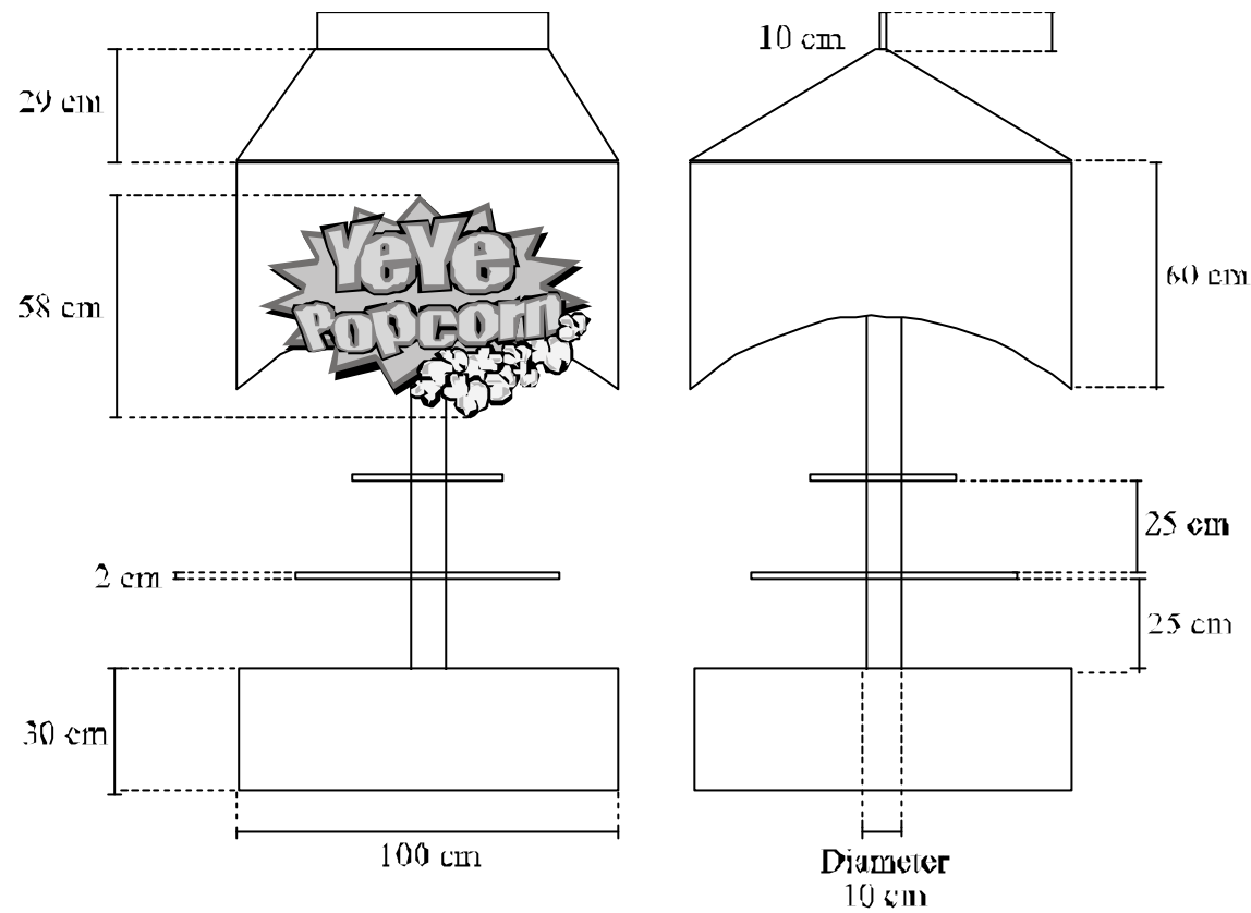
Gambar 6.36. Gambar Teknik Display Floor
