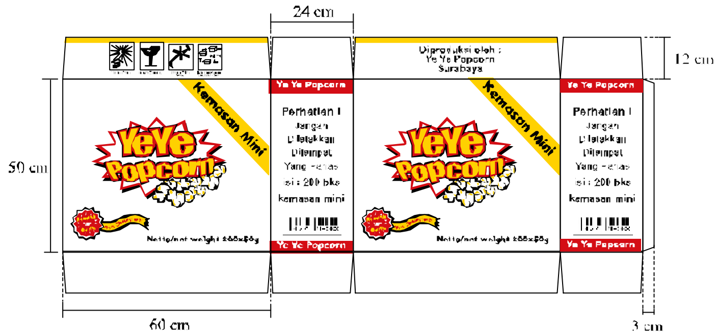
Gambar 6.10, Pattern Kemasan Sekunder Mini
